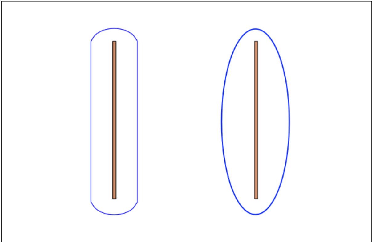
Figuur 6: conceptuele vergelijking tussen de invloedstraal voor de bemaling van een sleuf berekend door middel van de Formule van Edelman (links) en gesimuleerd in een grondwatermodel (rechts).
