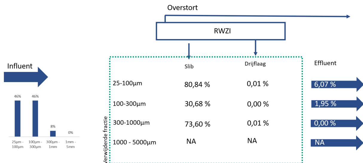
Figuur 14: Gedifferentieerde stofstoomanalyse (deeltjes) in een rioolwaterzuiveringsinstallatie in Grimbergen in een droge staalname periode op basis van deeltjesgrootte
