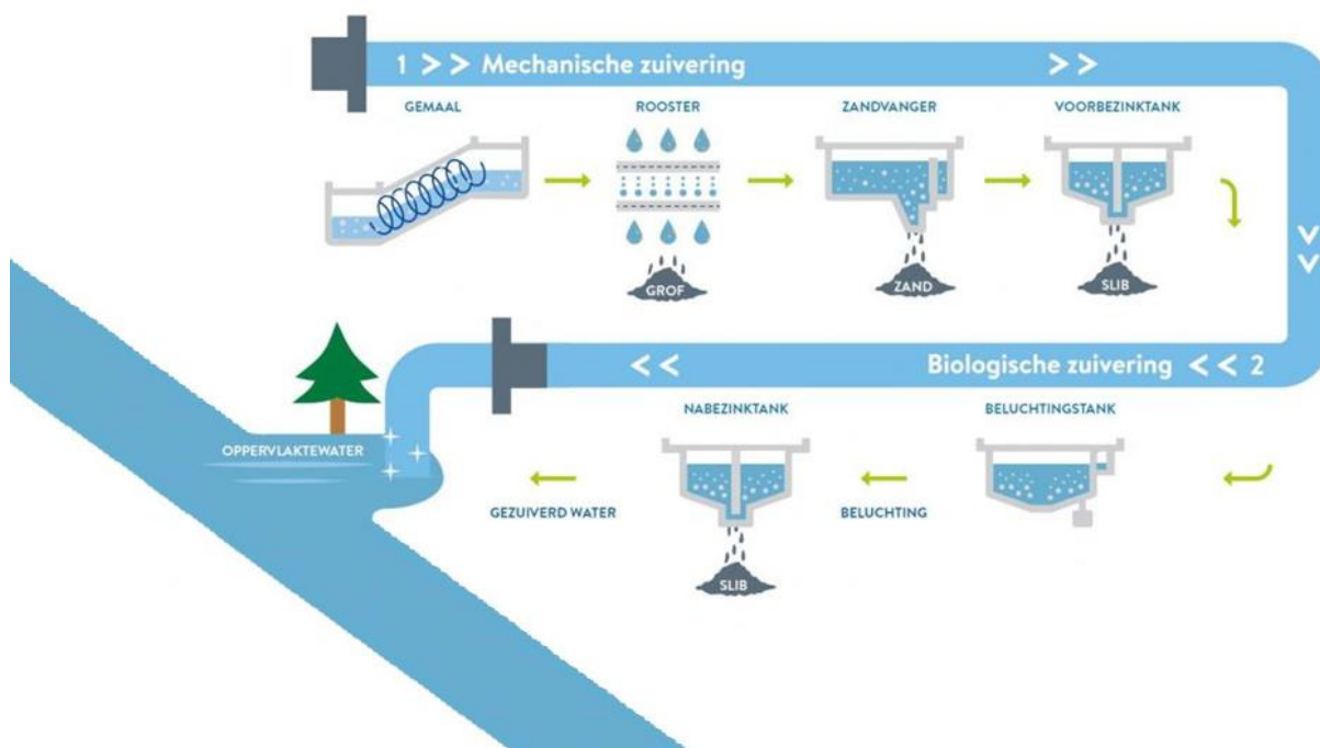
Figuur 1: Schematische voorstelling van de verschillende zuiveringsstappen in een rioolwaterzuiveringsinstallatie
