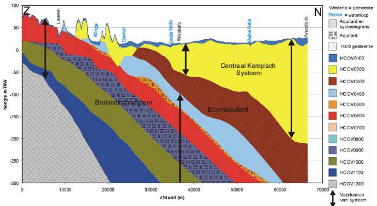
Profiel 2: grondwaterlagen tussen Arendonk (noorden van de provincie Antwerpen) en Leuven (zuiden van de provincie Vlaams-Brabant)
