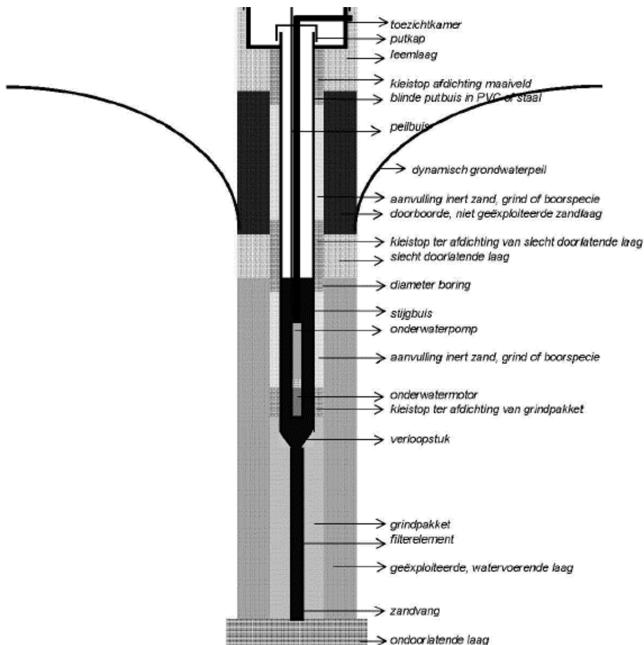
Figuur 6: opbouw van een grondwaterput volgens de code van goede praktijk (bijlage 5.53.1, titel II van de VLAREM)
