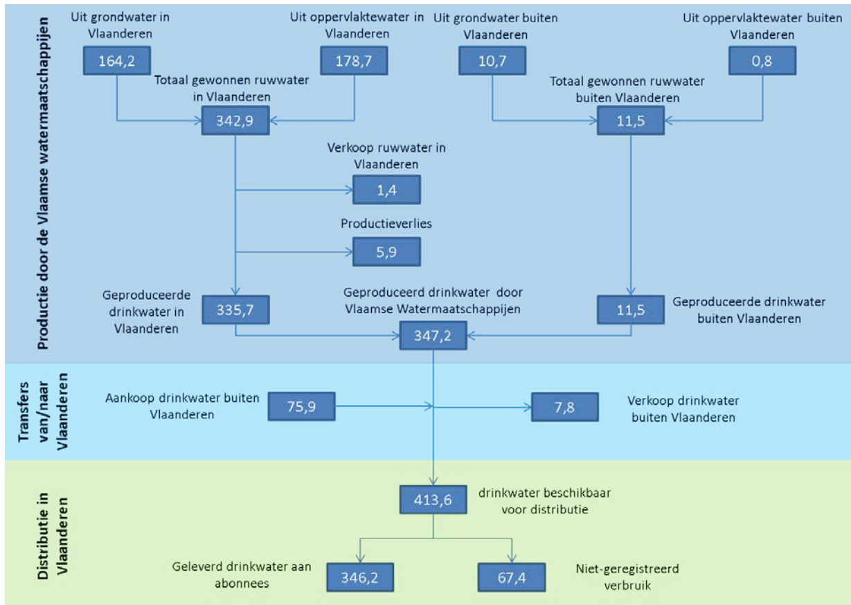
Figuur 2: Waterbalans 2012 (volumes uitgedrukt in miljoen m 3 ).
