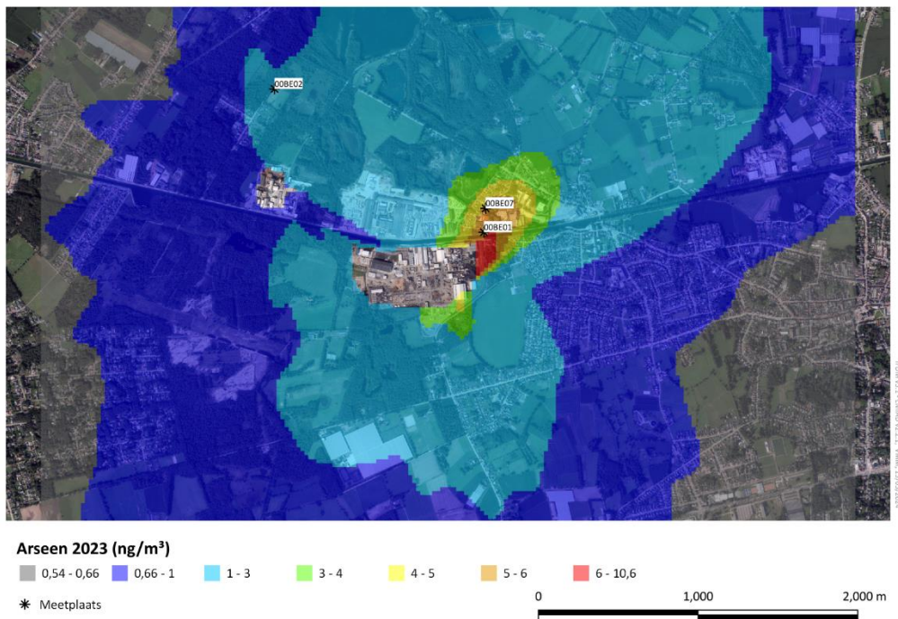
Figuur 3: Modellering arseen in 2023
